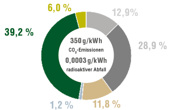
BUNDESDEUTSCHER STROMMIX
